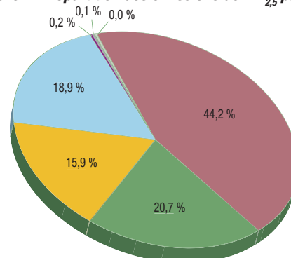
Figure 11 : répartition des émissions de PM 2,5 par secteur d'activité
